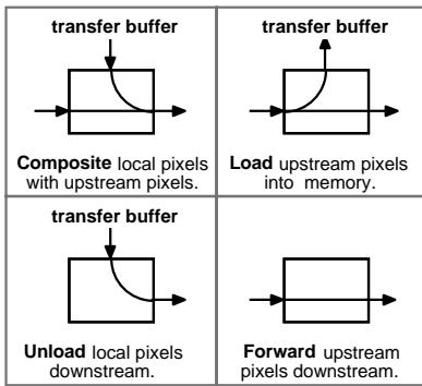
Figure 7: Compositor modes.
